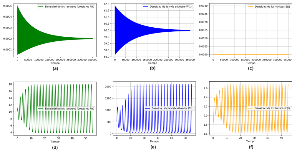
Figura 4. Las soluciones convergen ya sea al equilibrio P_1 o a una órbita periódica P^0 .
