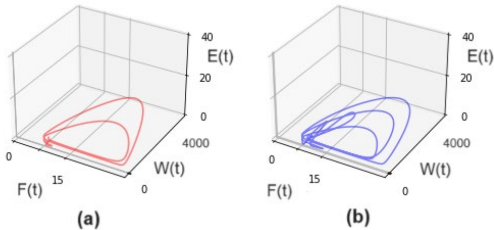
Figura 6. Atractor caótico
