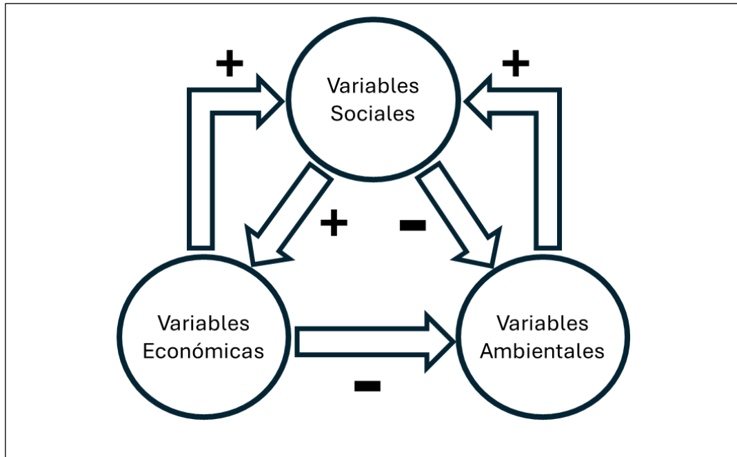
Figura 1. Efectos asociados a las interacciones entre las variables usadas en el modelo. La flecha describe el efecto positivo (+) o negativo (-) recibido por una variable desde la otra.
